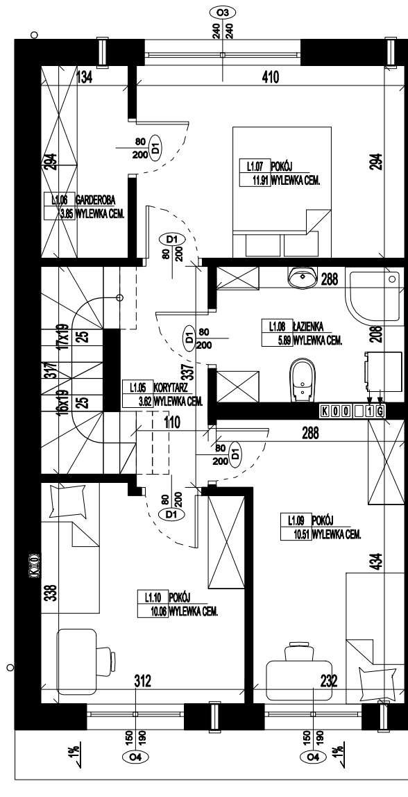
RZUT PIĘTRA LOKAL 1
