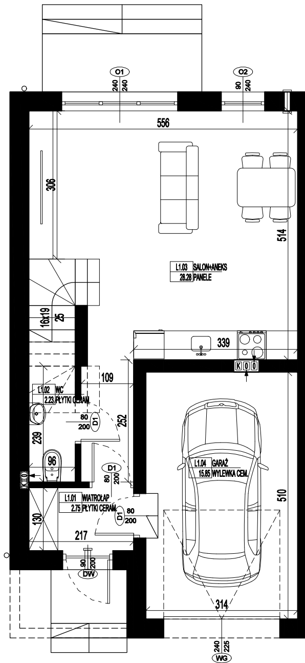
RZUT PARTERU LOKAL 1
